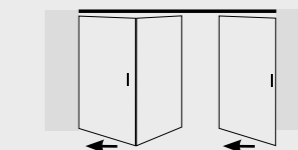
1 puerta plegable 2 hojas fijación lateral + 1 puerta pivotante 1 hoja fijación central
