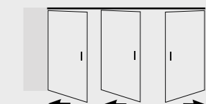
2 puertas pivotantes 1 hoja fijación lateral + 1 puerta pivotante 1 hoja fijación central
